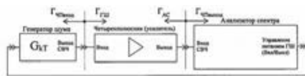
Рисунок 1б. Измерение суммарного коэффициента шума четырехполюсника в анализаторе спектра КШ сум
