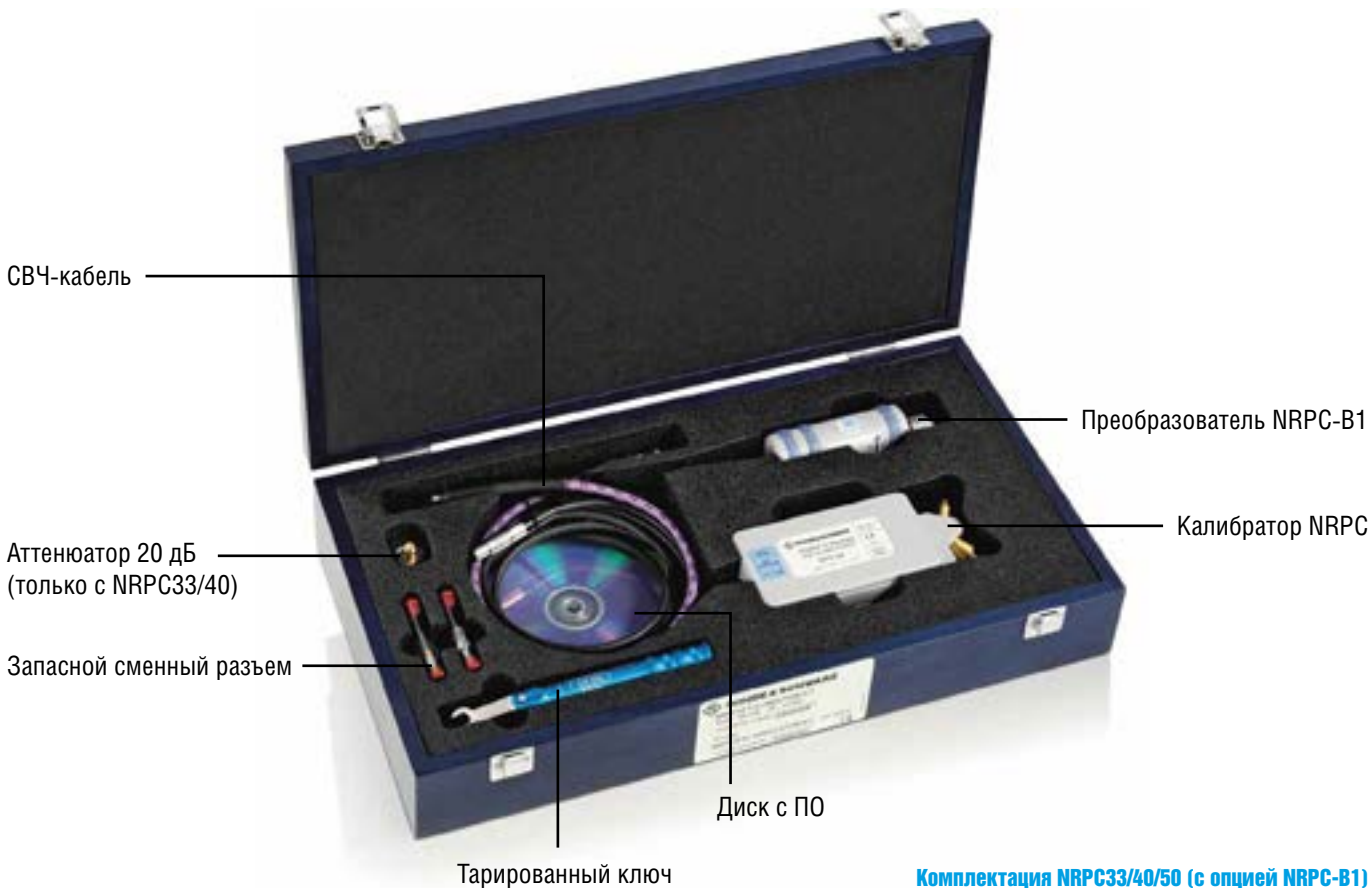
Комплектация NRPC33/40/50 (с опцией NRPC-B1)
